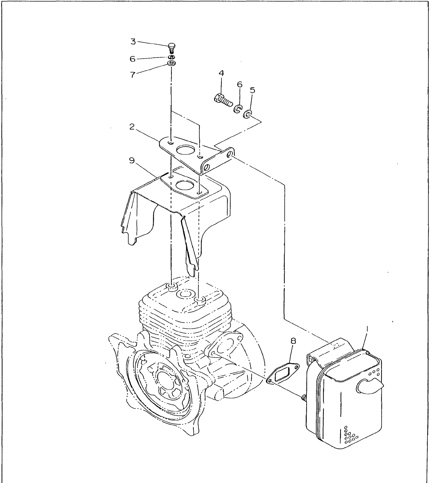
FIG. 3 MUFFLER
